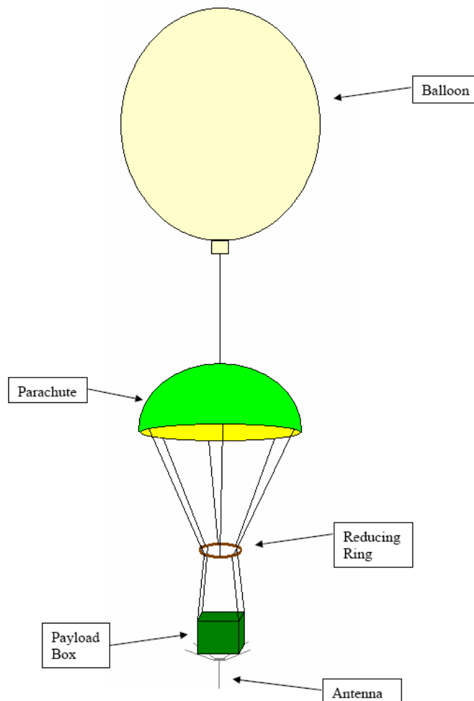
Figure 2: HAB Module
